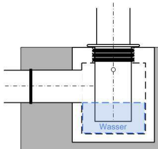
Type US (siphonné en bas)
