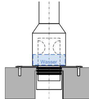
Type OS (siphonné en haut)
