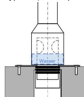
Typ OS (oben siphoniert)
