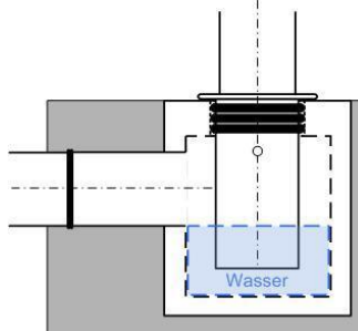
Unten siphoniert in Verbindung mit dem Bodenstück Nr. 2106
