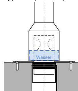
Oben siphoniert im Standrohr von Leer-/Überlauf integriert.
