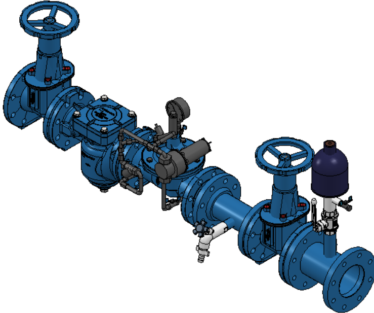
Type 1400, installée comme vanne de maintien pression
